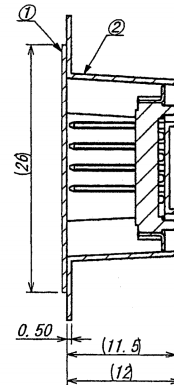
SECT A-A
