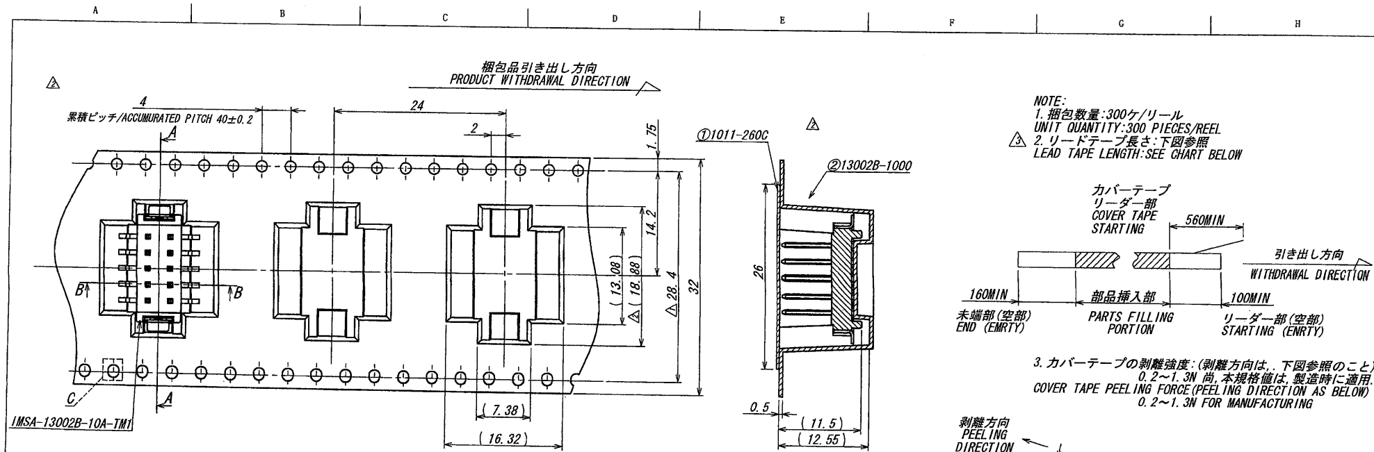
SECT A-A
