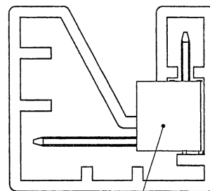
① ストッパー位置 STOPPER POSITION
