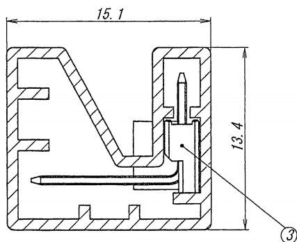
SECT A-A
