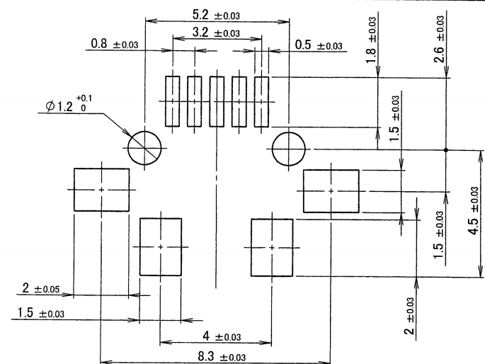
推獎基板寸法 RECOMMEND PCB LAYOUT
