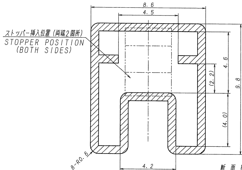
断面拡大図 SECT. DETAILS
