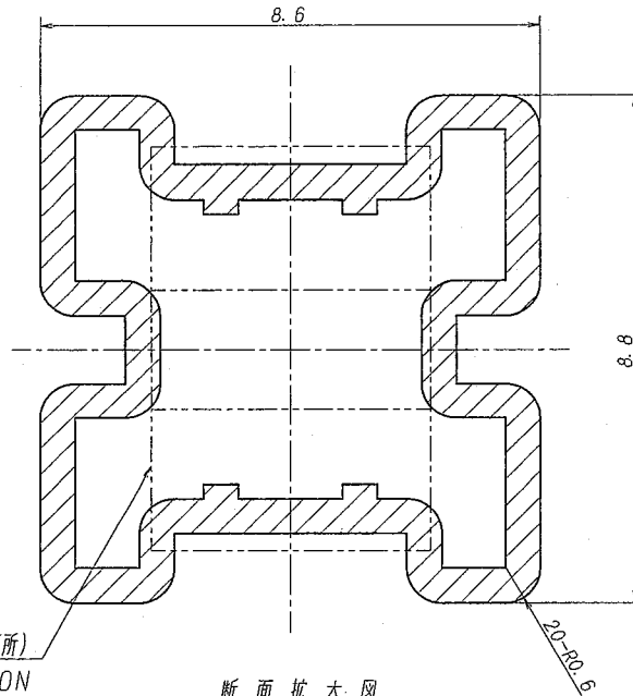
断面拡大図 SECT. DETAILS
