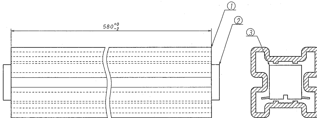
断面拡大図 SECT. DETAILS
