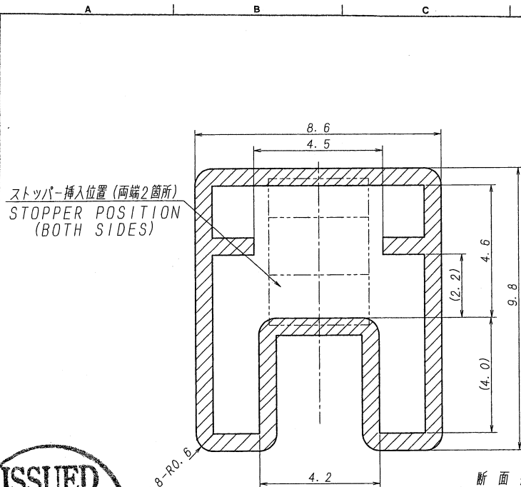
断面拡大図 SECT. DETAILS
