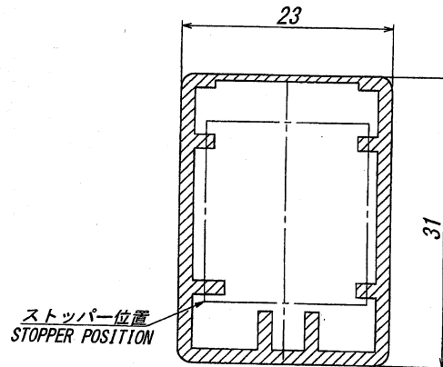
断面拡大図 SECT. DETAIL
