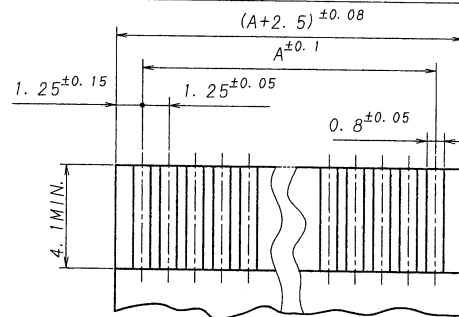
FPC/メンブレン推奨寸法
