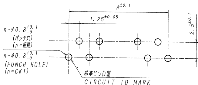
取付基板寸法 (コネクタ搭載側)
