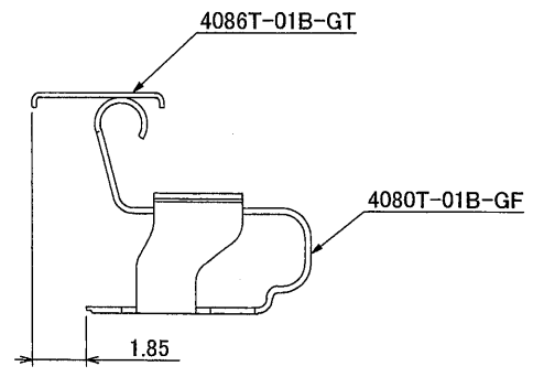
Fig.1 嵌合位置/MATE POSITION
