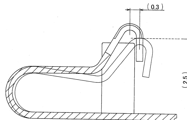
SECT A-A
