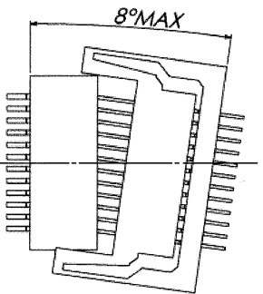
誘い込み時の角度 Guiding angle
